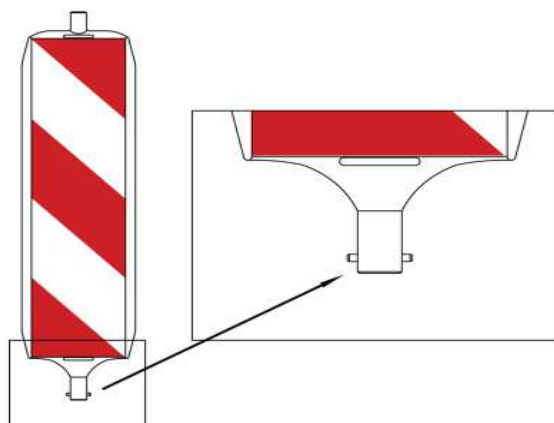
Пример могуће монтаже вертикалне запреке - монтажни систем „окрени и закључај“
