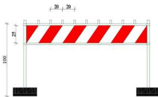
Чеона запрека VII-1.1 - лева
